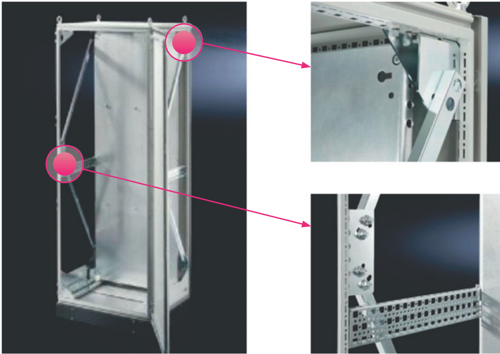
Abbildung 2: Erdbebenerweiterungszubehör für den TS 8
