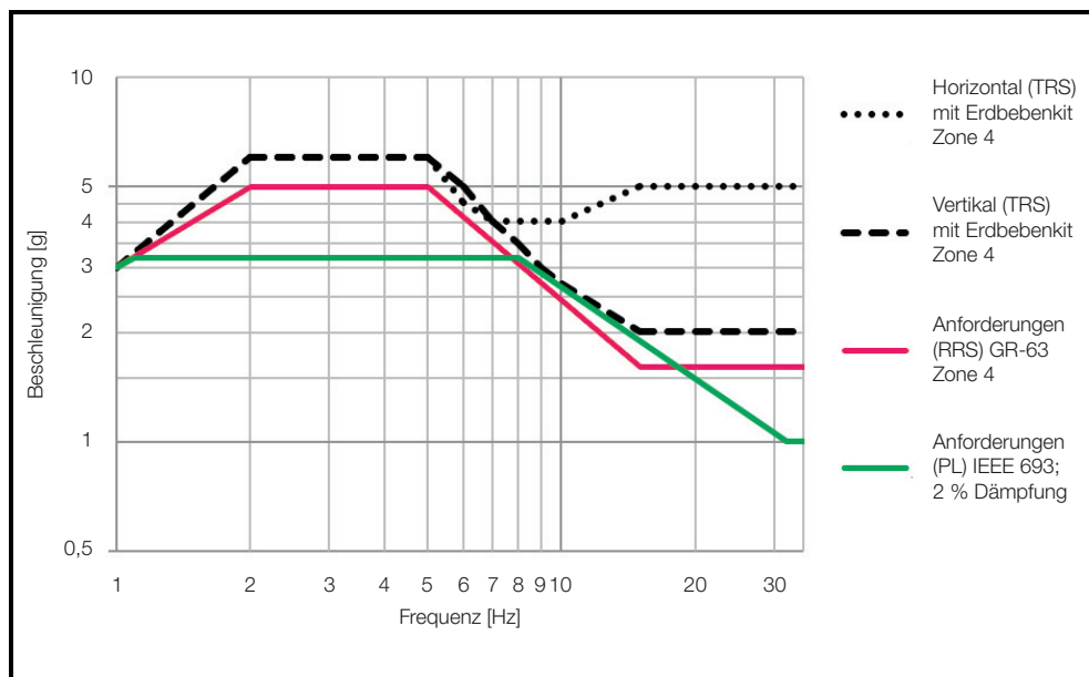
Abbildung 1: Beschleunigung-Frequenz-Diagramm
